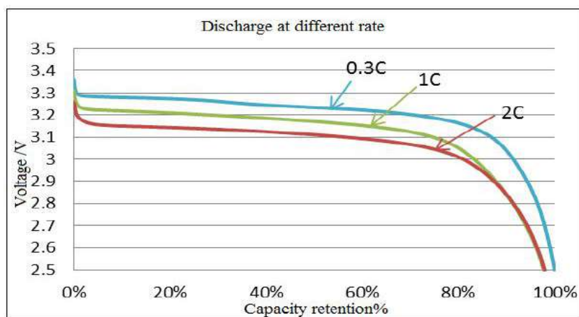
图 1. SP-LFP-100F I 常温放电曲线
