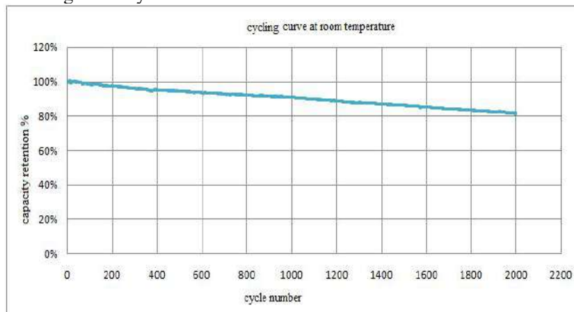
图 3. SP-LFP-100F I 1C 常温循环曲线
