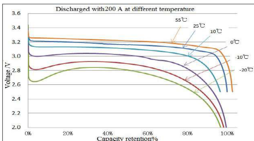
图 2. SP-LFP-100F I 不同温度放电曲线
