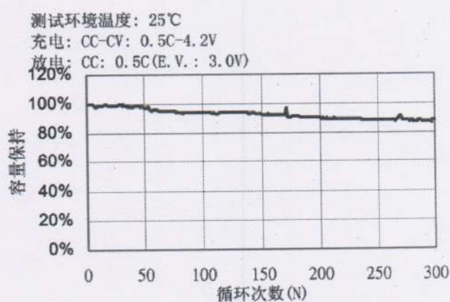
循环特性
