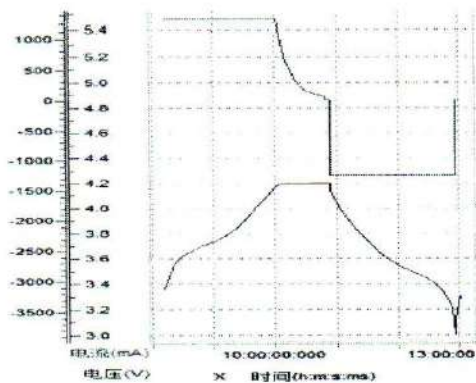
充放电曲线
