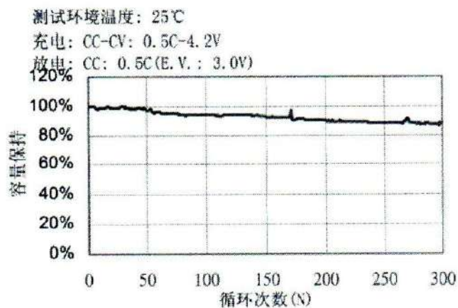
循环特性
