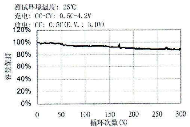
循环特性
