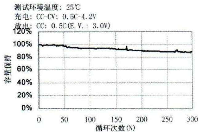
循环特性
