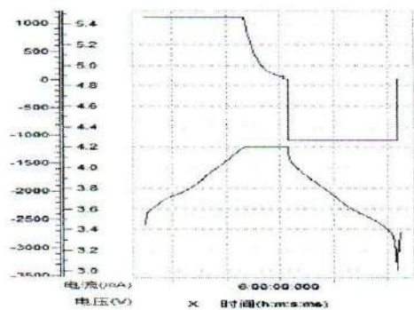
充放电曲线
