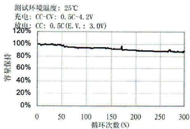
循环特性
