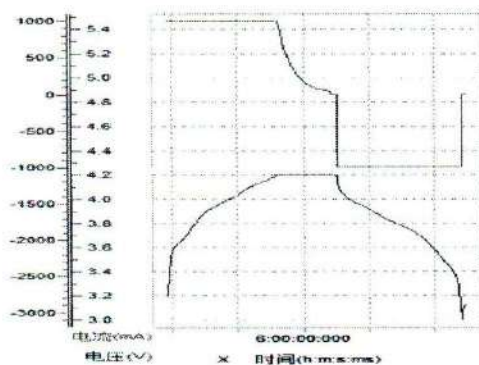
充放电曲线
