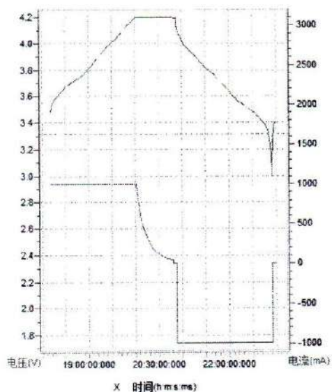
充放电曲线
