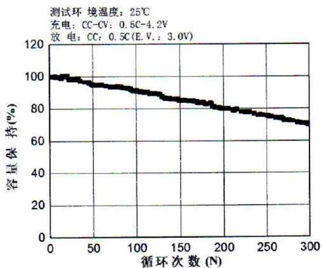
循环特性
