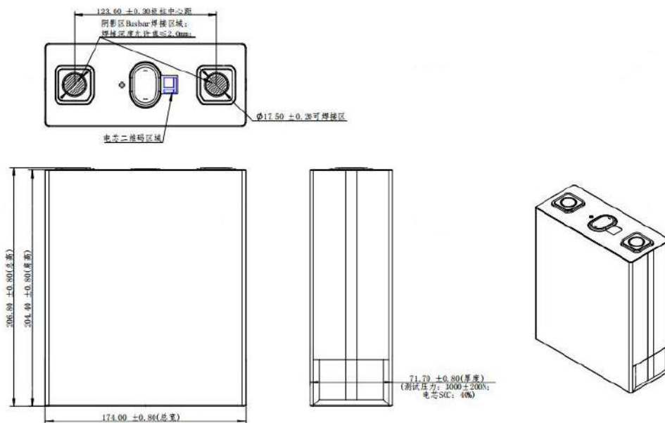
图 7.1 电池尺寸/mm
