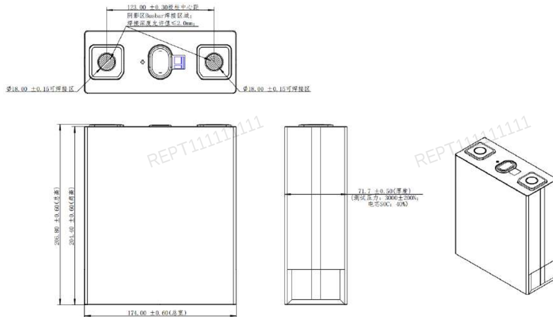
图 7.1 电池尺寸/mm
