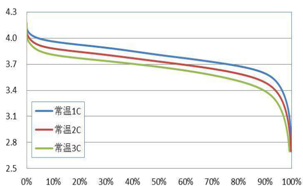
1833-10Ah常温倍率曲线
