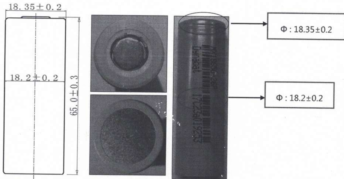
MX18650-26P 外形尺寸图
