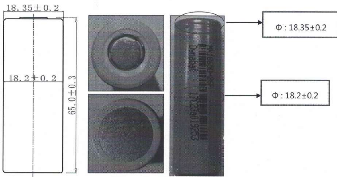
MX18650-26P 外形尺寸图
