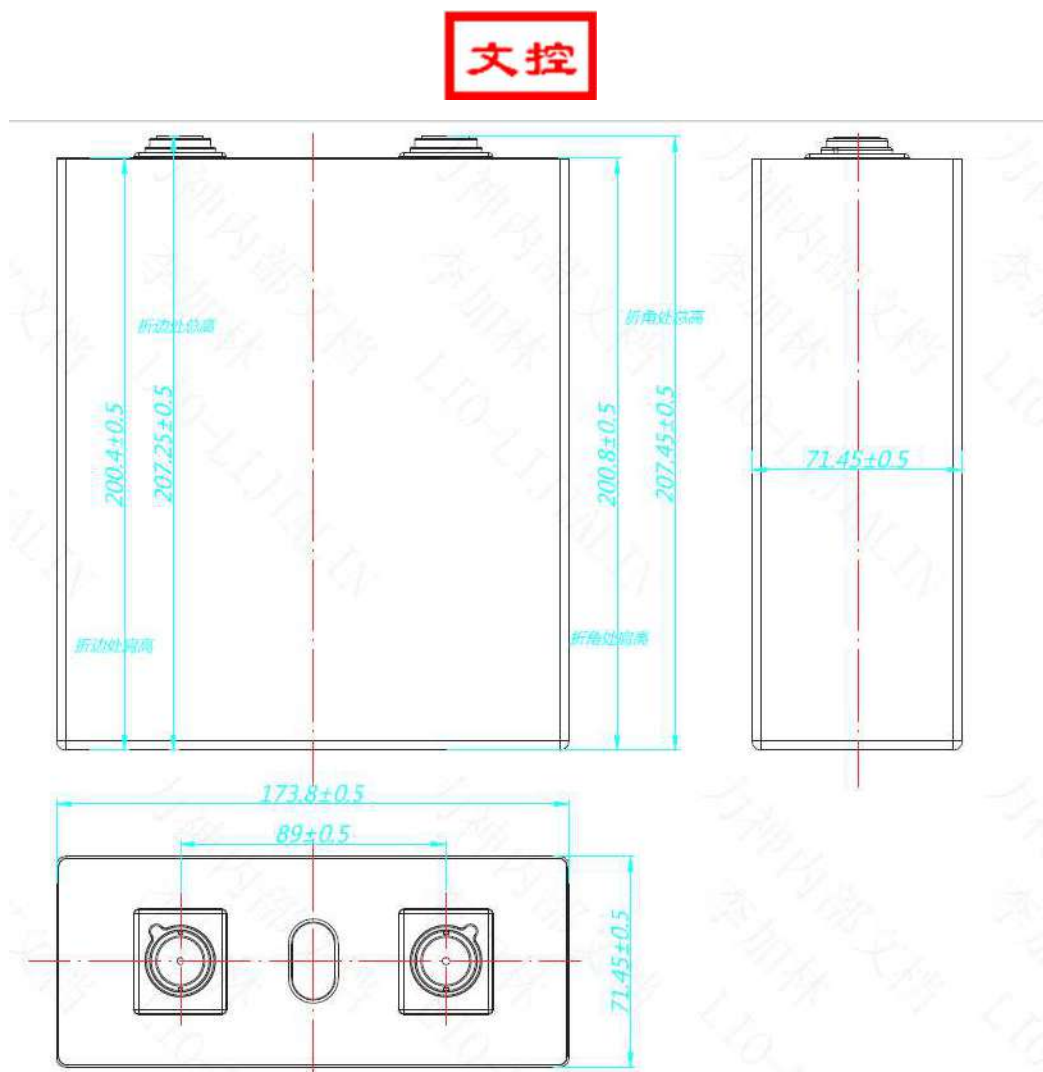
图 1 电池外形图
