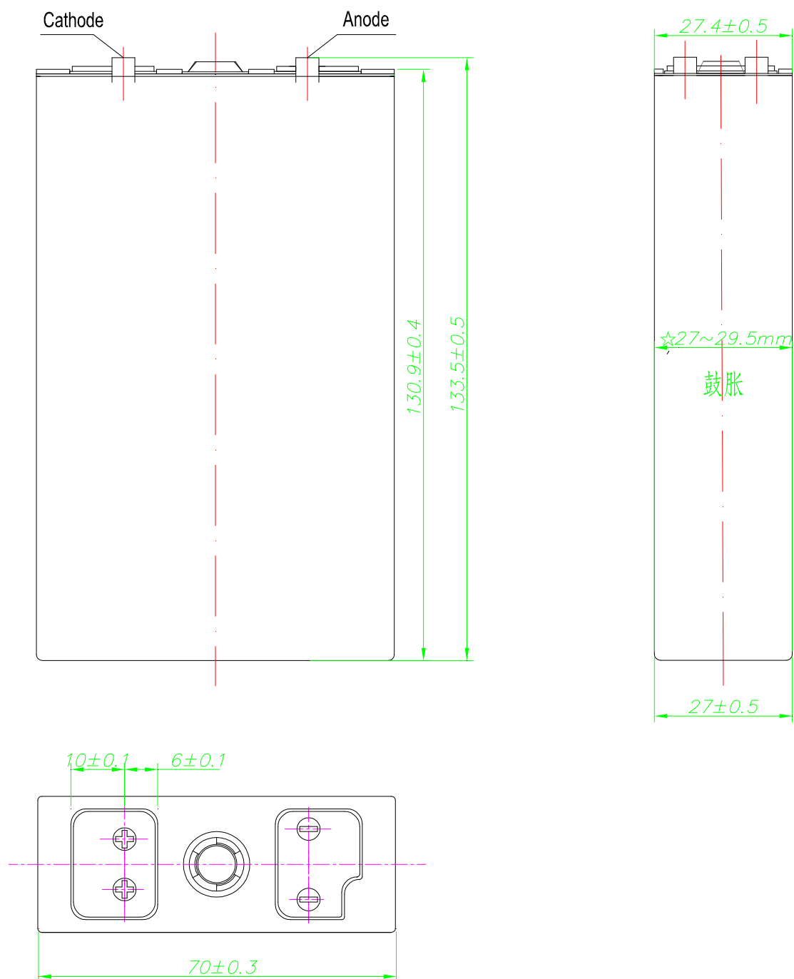
图 1 电池外形图
