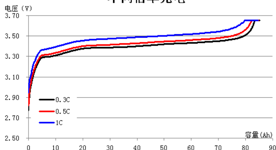
不同倍率充电
