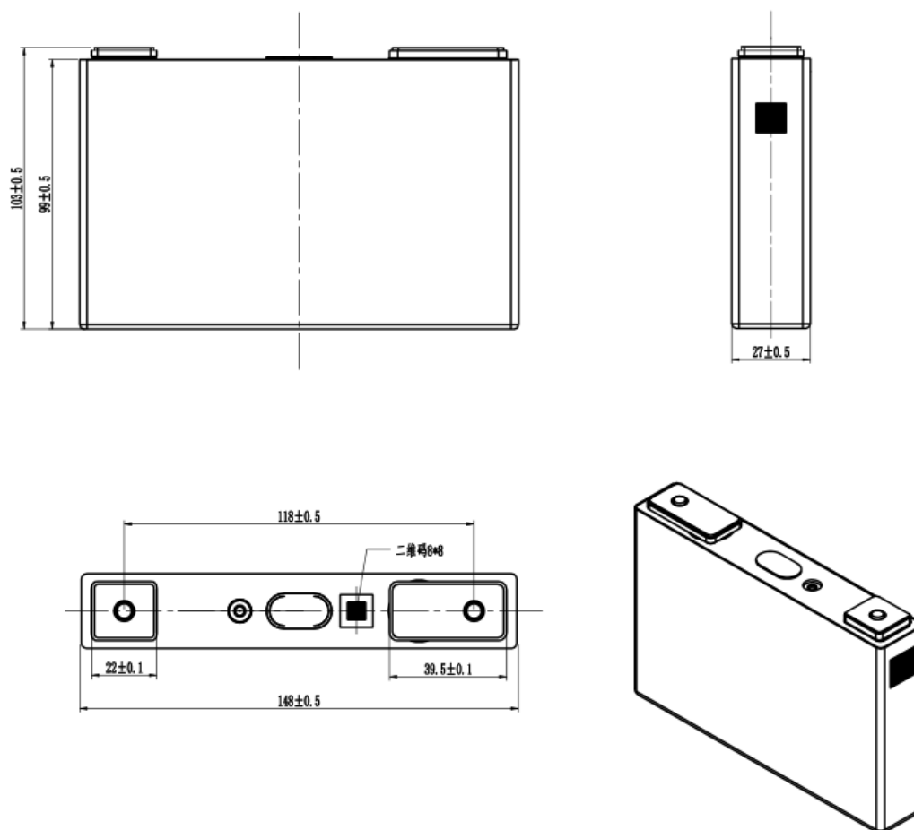
图 A. 1 电池尺寸图
