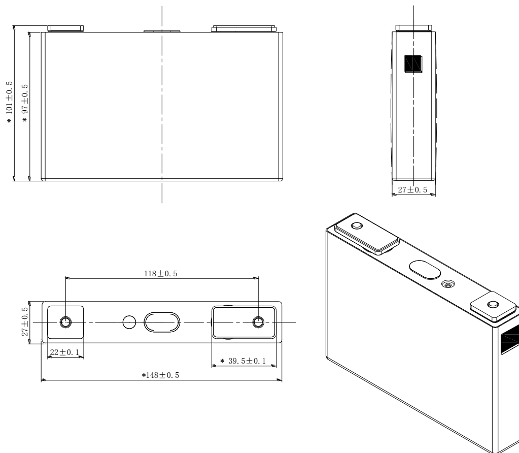
图 A.1 电池尺寸图
