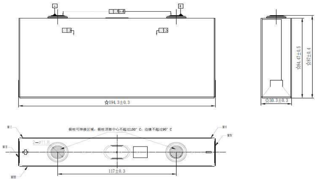
二维图纸
