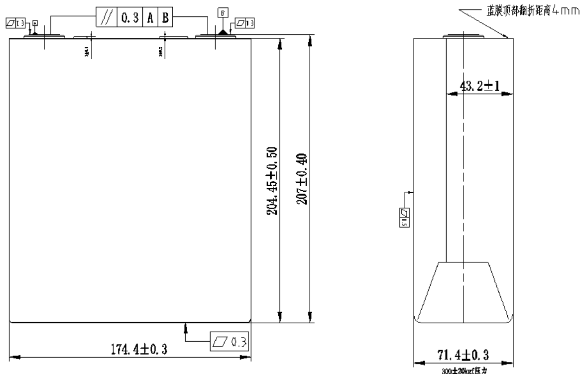
二维图纸
