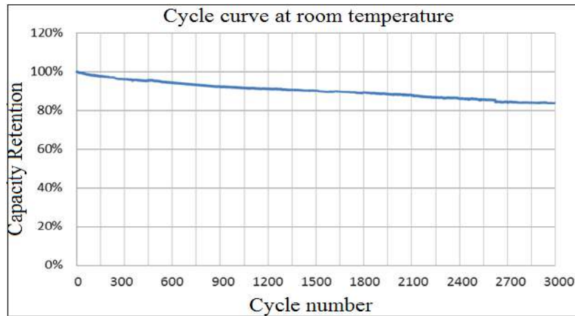
图 3. L148F20D 常温循环曲线
