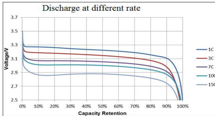
图 1. L148F20D 常温放电曲线
