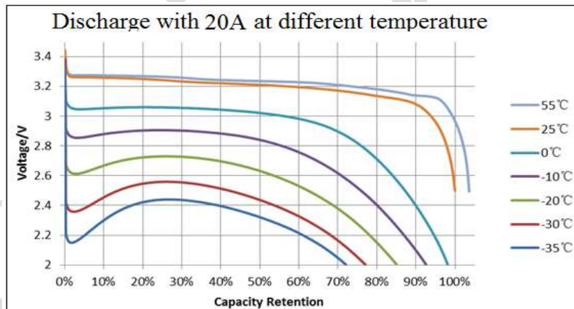
图 2. L148F20D 不同温度放电曲线
