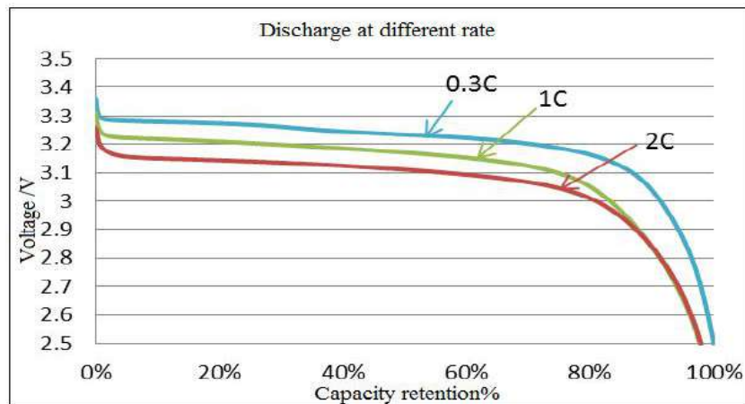
图 1. SE200FC 常温放电曲线
