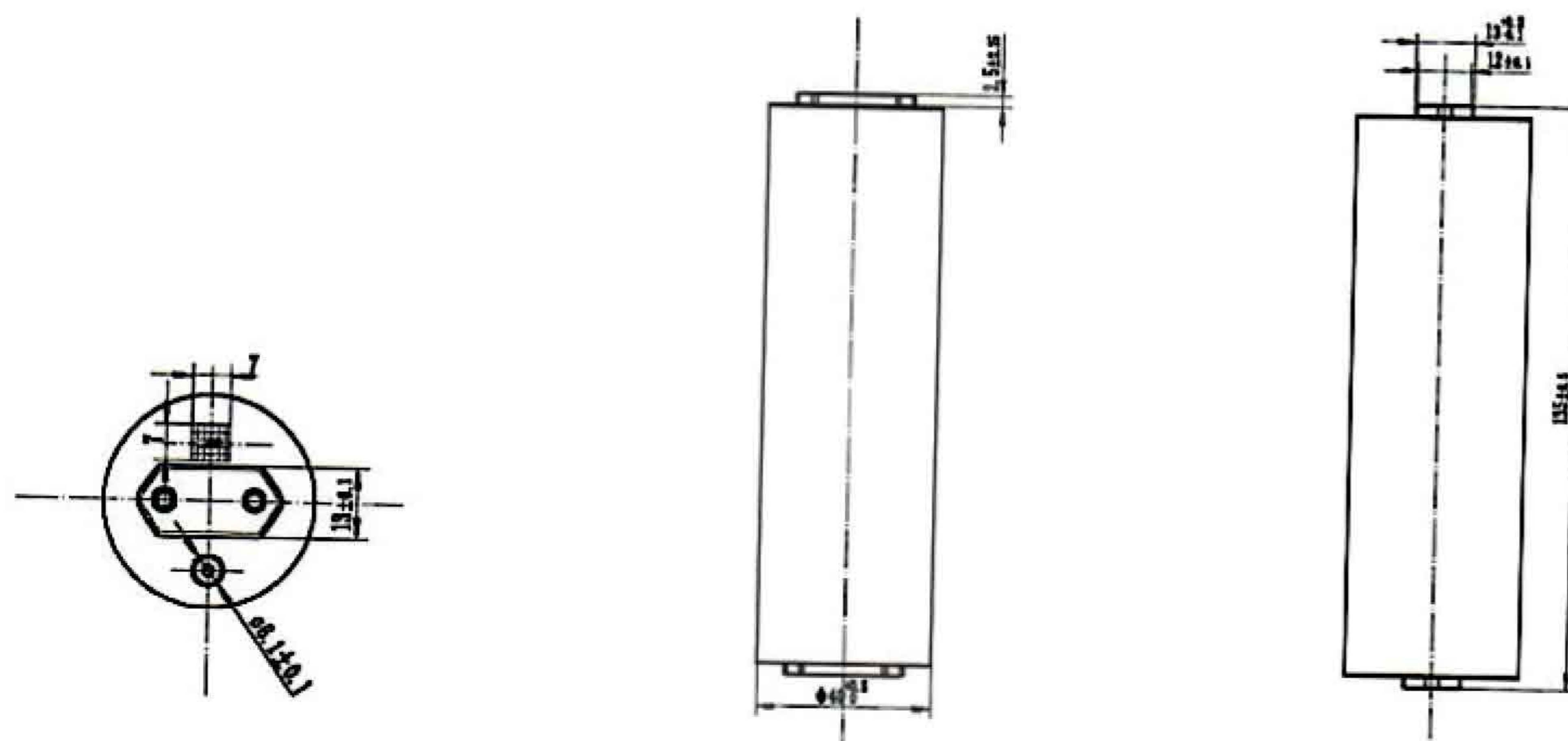
图A 电池图片和外形尺寸
