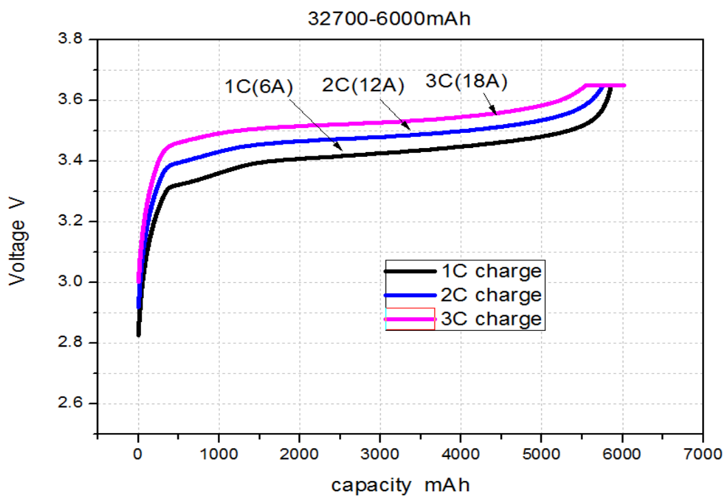
6.0Ah 磷酸铁锂系电池不同倍率充电曲线 Different rate charge curve of 6.0Ah LiFePO 4 Cell
