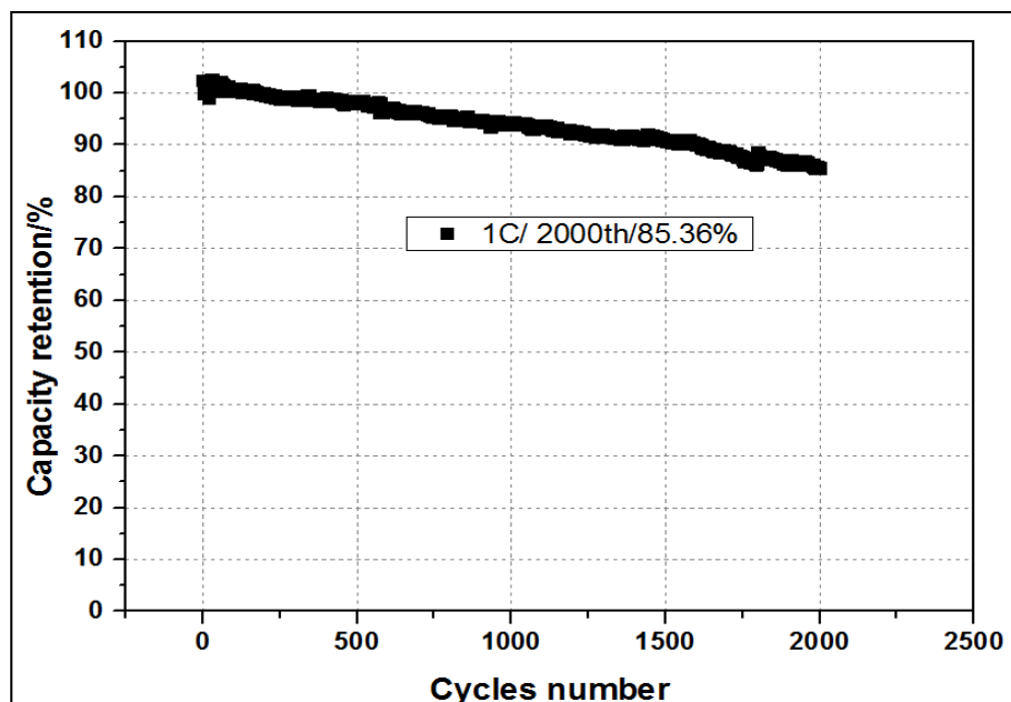
6.0Ah 磷酸铁锂系电池循环曲线 Cycling curve of 6.0Ah LiFePO 4 cell
