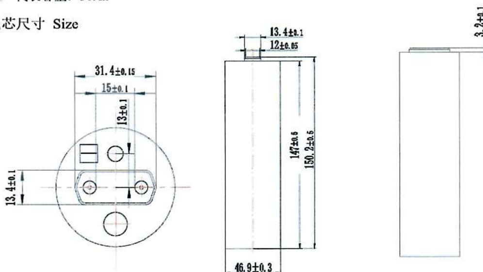
图A 电池图片和外形尺寸
