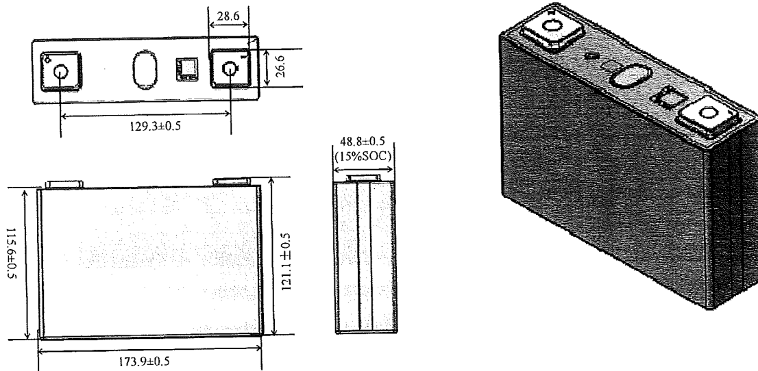
图1 电芯尺寸 (含蓝膜+顶贴片+底贴片)
